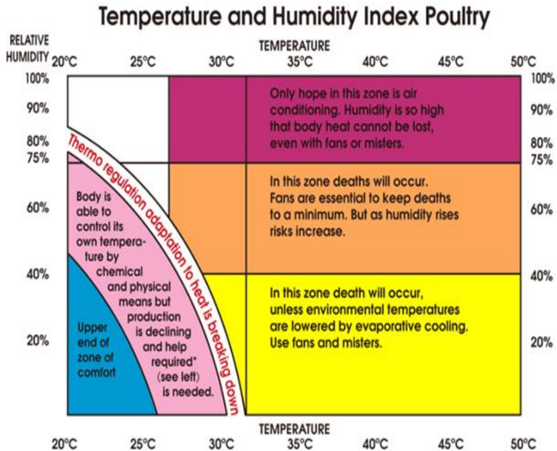
Figura 7 - La figura mostra le aree di comfort termico per le specie avicole, in base a temperatura e umidità relativa e le soglie al di sopra delle quali gli animali iniziano a sviluppare stress da caldo
